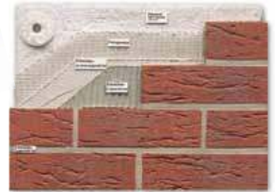
Классическая система облицовки фасада по сетке и утеплителю пенопласт (вспененный пенополистерол)
